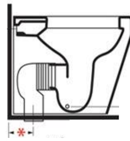
NUOVO VASO FILO PARETE SU VECCHIO IMPIANTO
